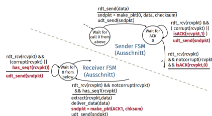
Abbildung 15: RDT 2.2 Zustandsautomat
