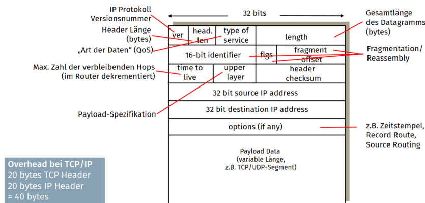
Abbildung 31: IPv4 Datagram format
