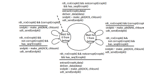
(b) RDT 2.1 Zustandsautomat Empfänger
