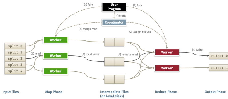
Abbildung 78: Google Map & Reduce Original Architektur
