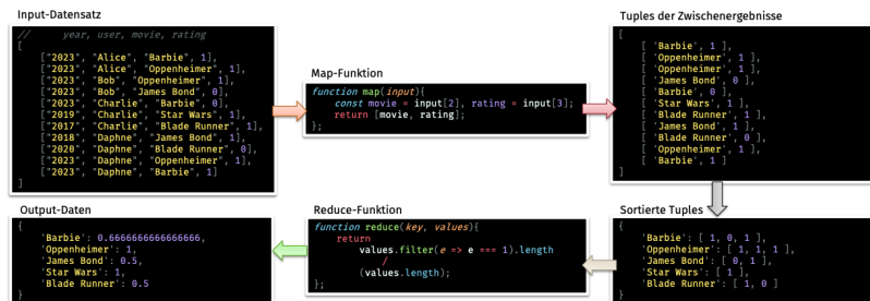
Abbildung 76: Map & Reduce Programmieren Beispiel
