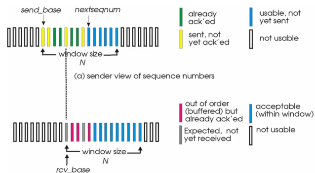
Abbildung 18: Selective Repeat
