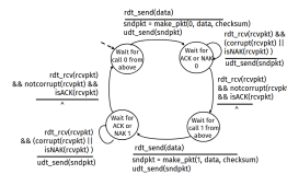
(a) RDT 2.1 Zustandsautomat Sender
