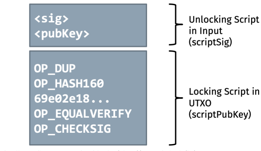
Abbildung 91: Bitcoin Transaktion Beispiel
