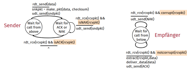
Abbildung 13: RDT 2.0 Zustandsautomat
