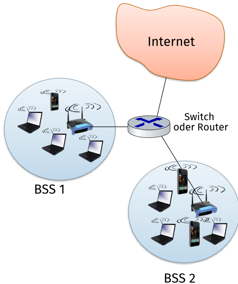
Abbildung 55: WLAN Architektur
