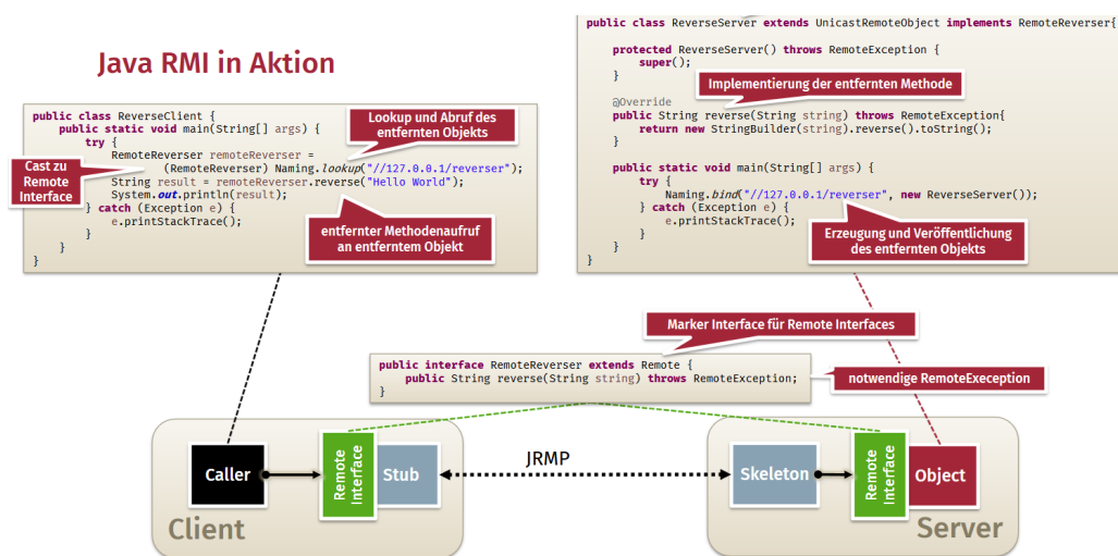
Abbildung 69: Java RMI in Aktion
