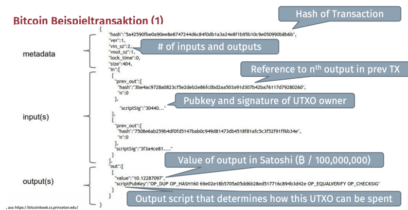
Abbildung 90: Bitcoin Transaktion Beispiel
