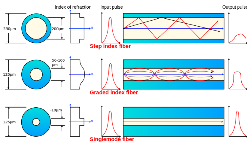
Abbildung 50: Glasfaser
